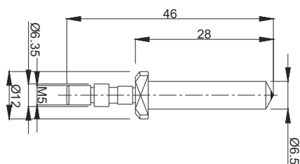
Reicherter Indenter
