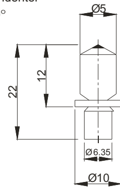
Reicherter Indenter
